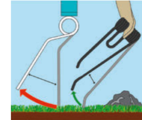
Suuren joustavuutensa ansiosta laahaavat Fendt Performance-piikit voivat myös välttää esteitä paljon helpommin kuin perinteiset piikit. Piikkien rikkoutuminen ei ole ongelma Lotuksessa.
