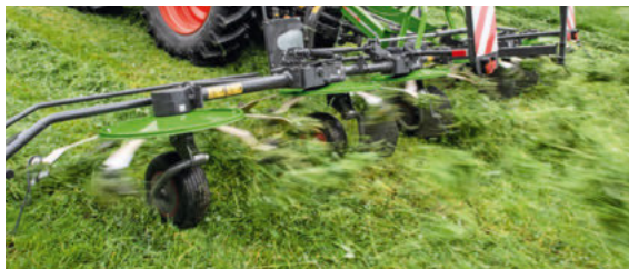
Kiertymisenestojärjestelmä estää satoa kiertymästä pyörän akselin ympärille.
